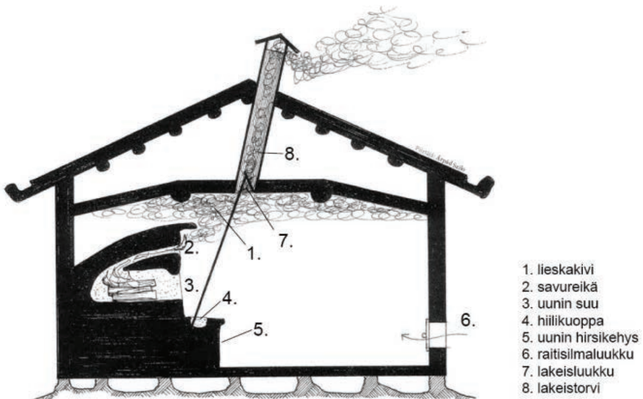
Savutuvan poikkileikkaus lämmitysjärjestelmän keskeisten osien kohdalta. Kuva Árpád Sálón diplomityöstä 4 .
